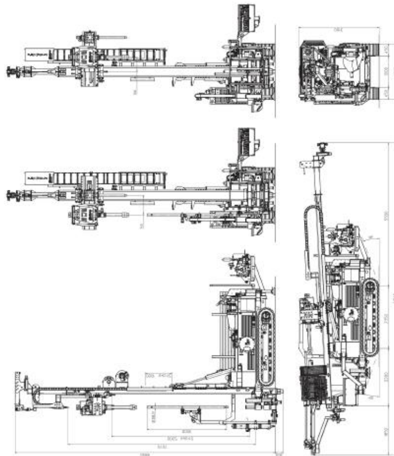
Fig.25 - Misure d'ingombro Fig.25 - Overall dimension
